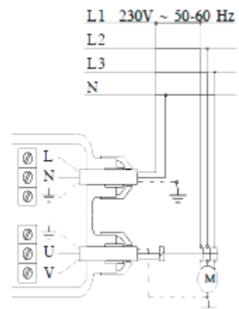
3-vaihemoottorit kytkentä
